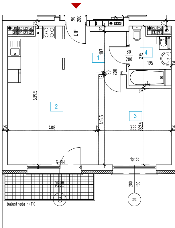
RZUT MIESZKANIA 1:100
