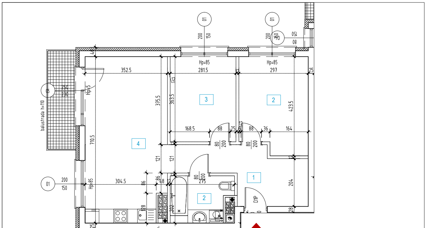
RZUT MIESZKANIA 1:100
