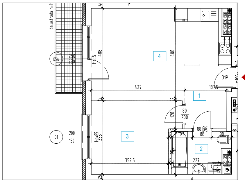
RZUT MIESZKANIA 1:100
