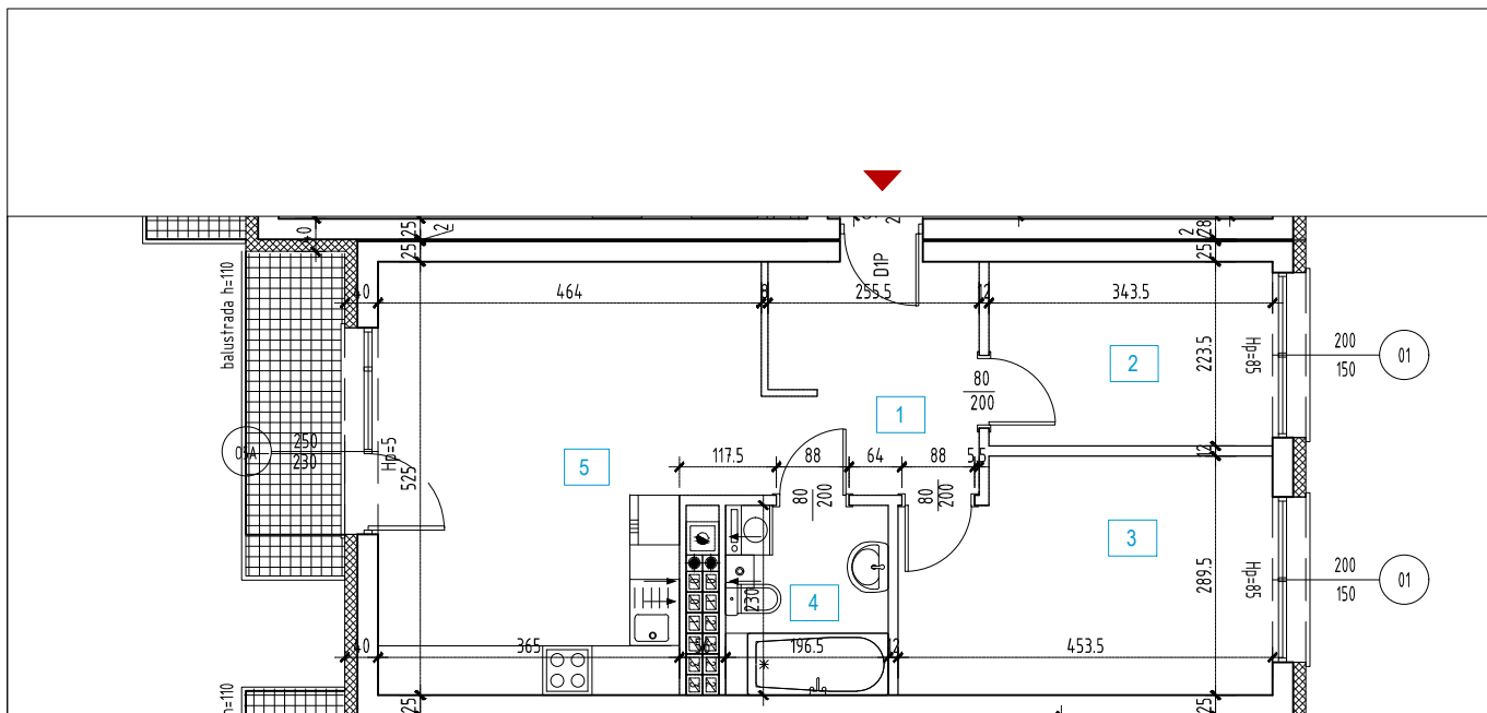
RZUT MIESZKANIA 1:100
