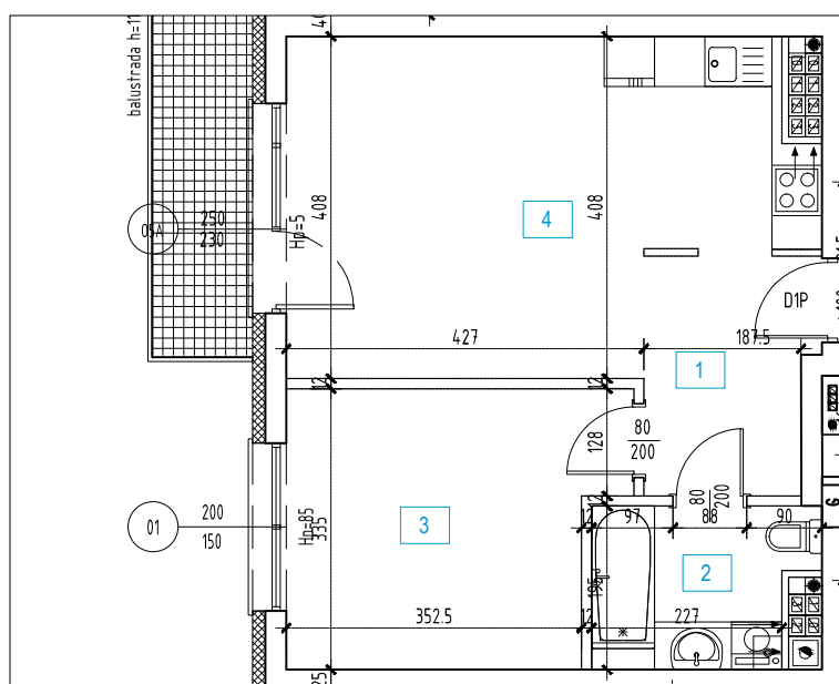
RZUT MIESZKANIA 1:100
