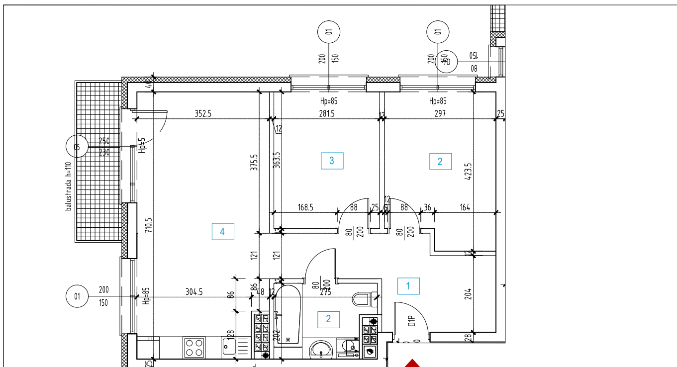
RZUT MIESZKANIA 1:100
