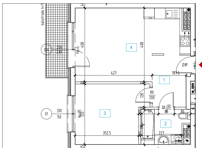
RZUT MIESZKANIA 1:100
