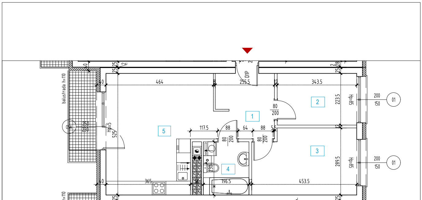
RZUT MIESZKANIA 1:100
