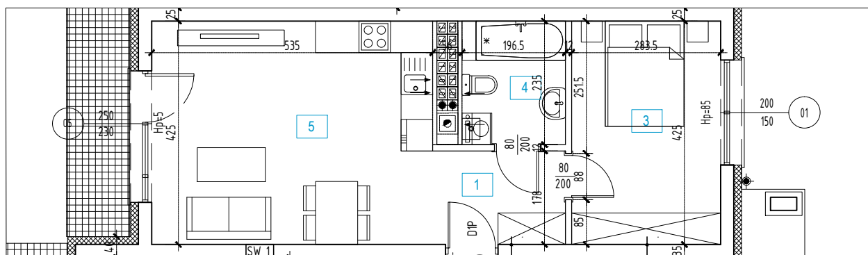
RZUT MIESZKANIA 1:100
