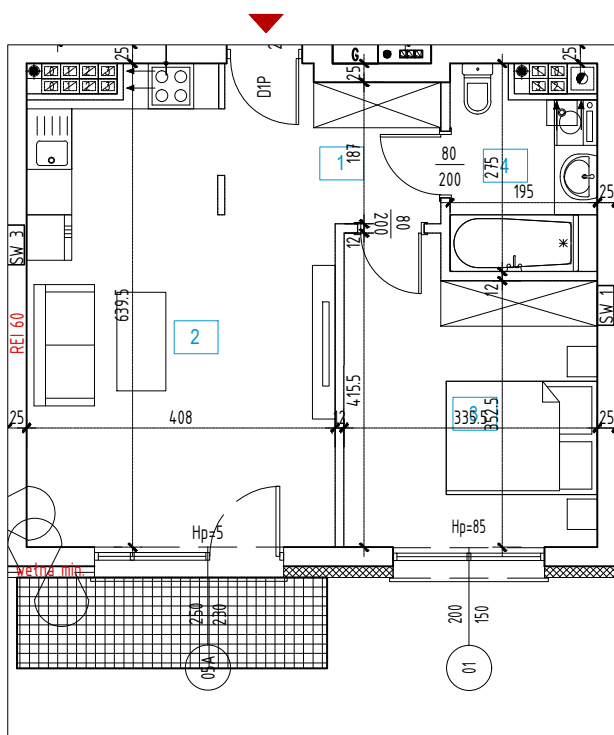
RZUT MIESZKANIA 1:100
