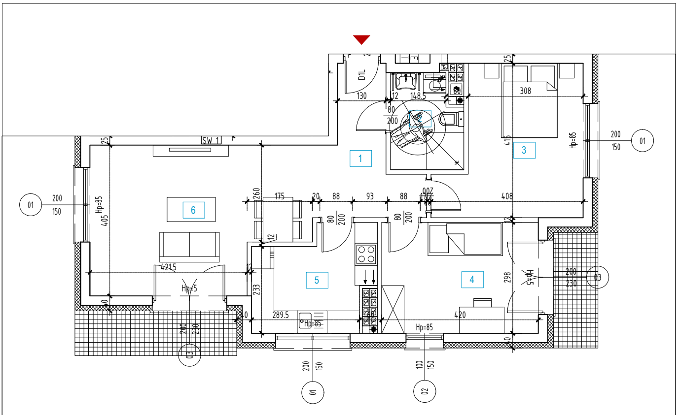
RZUT MIESZKANIA 1:100
