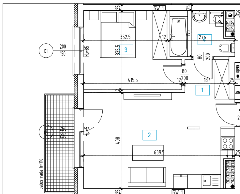
RZUT MIESZKANIA 1:100
