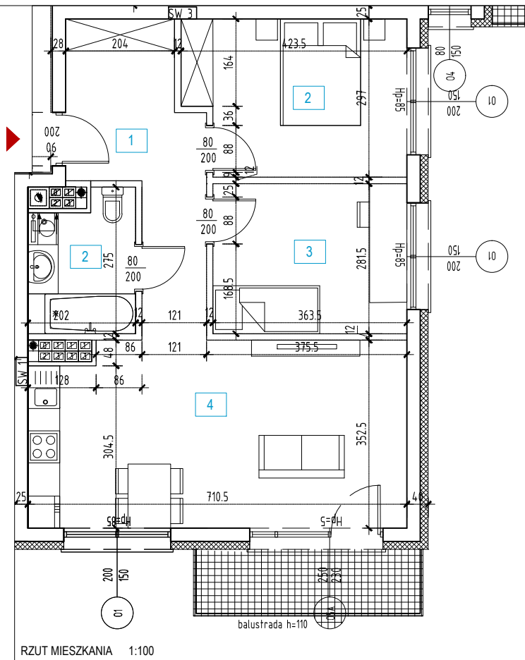
RZUT MIESZKANIA 1:100
