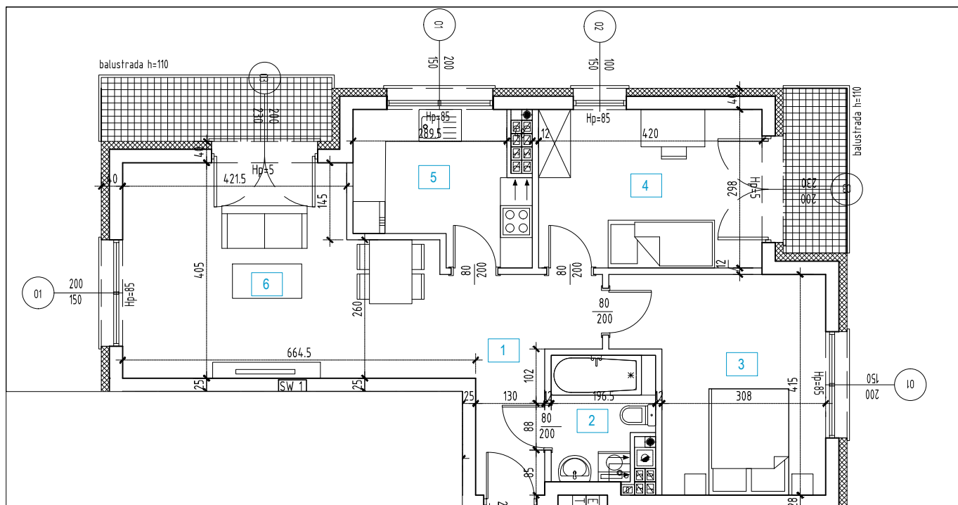
RZUT MIESZKANIA 1:100
