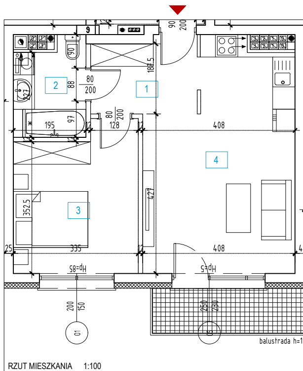
RZUT MIESZKANIA 1:100
