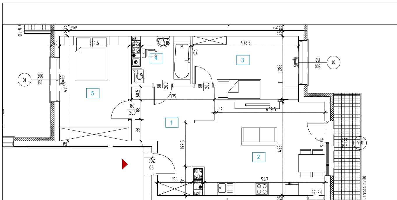
RZUT MIESZKANIA 1:100
