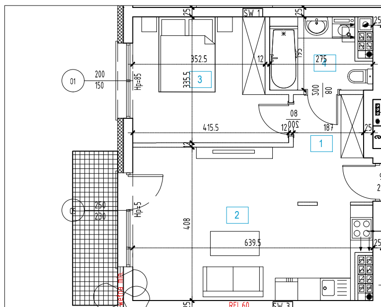
RZUT MIESZKANIA 1:100
