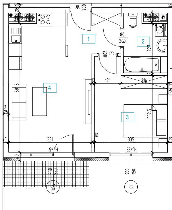
RZUT MIESZKANIA 1:100
