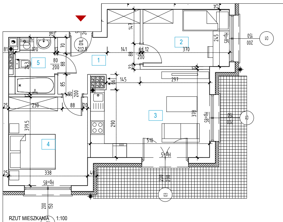
RZUT MIESZKANIA 1:100
