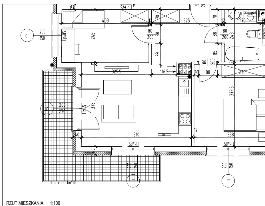
RZUT MIESZKANIA 1:100
