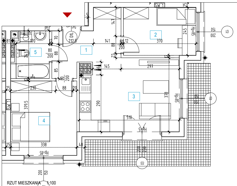
RZUT MIESZKANIA 1:100
