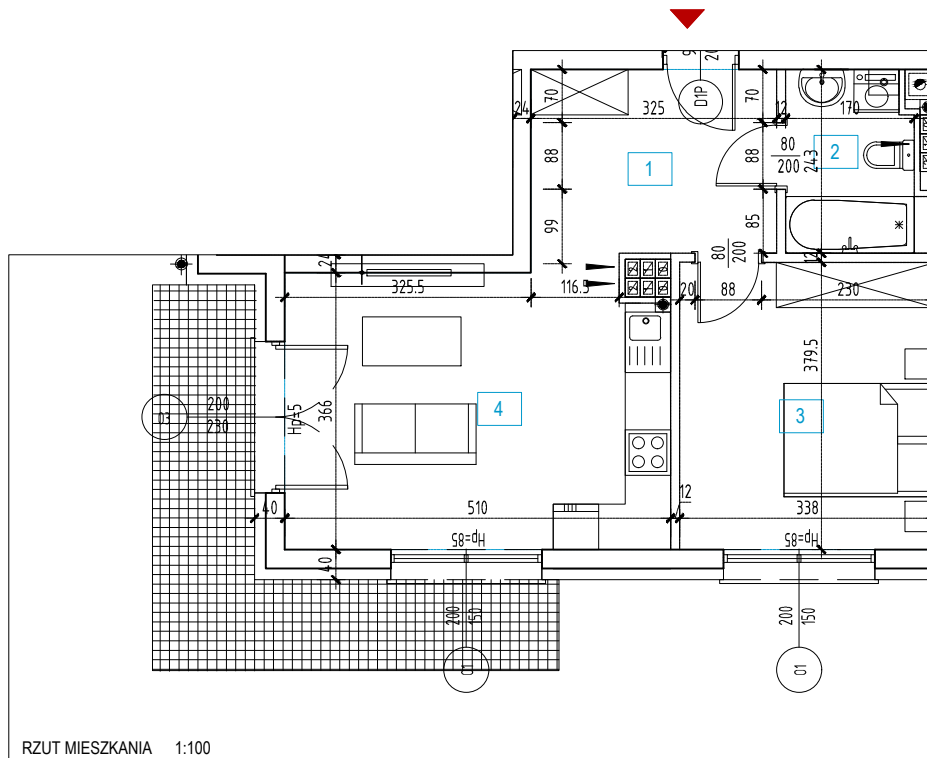
RZUT MIESZKANIA 1:100
