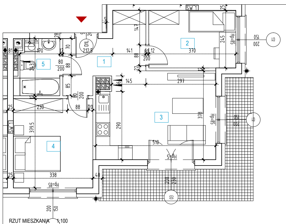
RZUT MIESZKANIA 1:100
