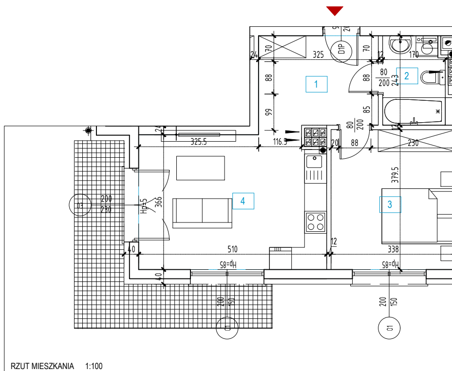
RZUT MIESZKANIA 1:100
